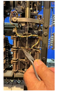
Hebdrehwähler- Nahaufnahme mit Werkzeug
